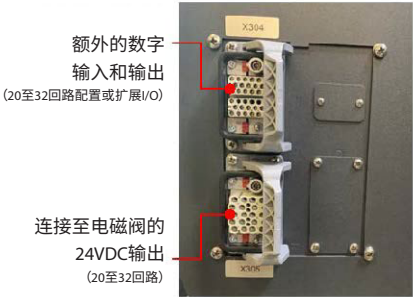
用于20至32回路配置或扩展I/O选配功能的额外连接器
