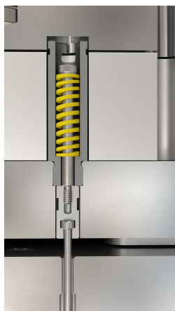
阀针打开与系统 接合
