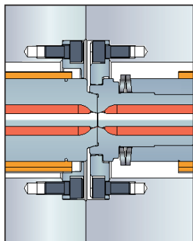
锥形阀针关断
