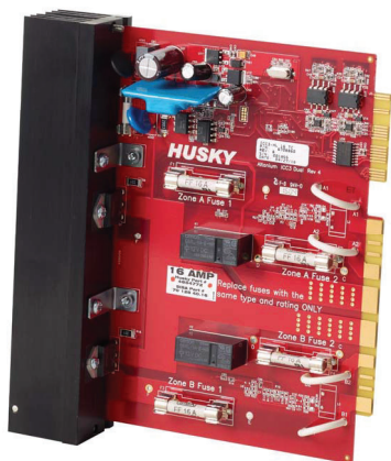
HL 系列 2z @ 16A 卡
